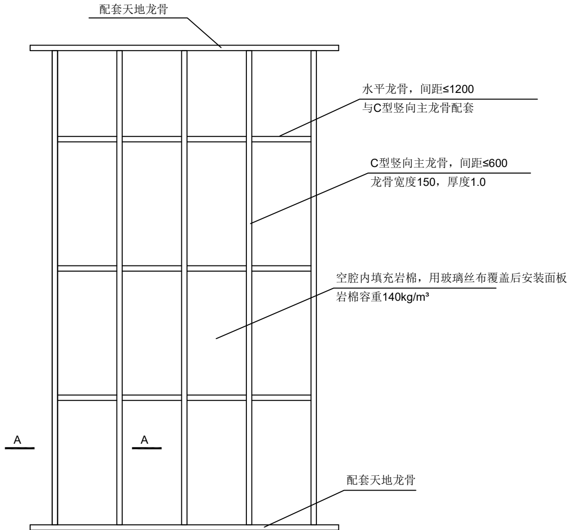
轻钢龙骨水泥板墙大样图
