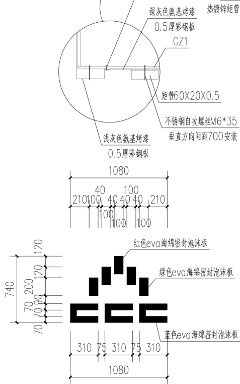
3C标志大样图
