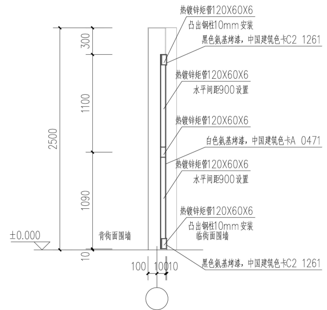
2-2剖面图
