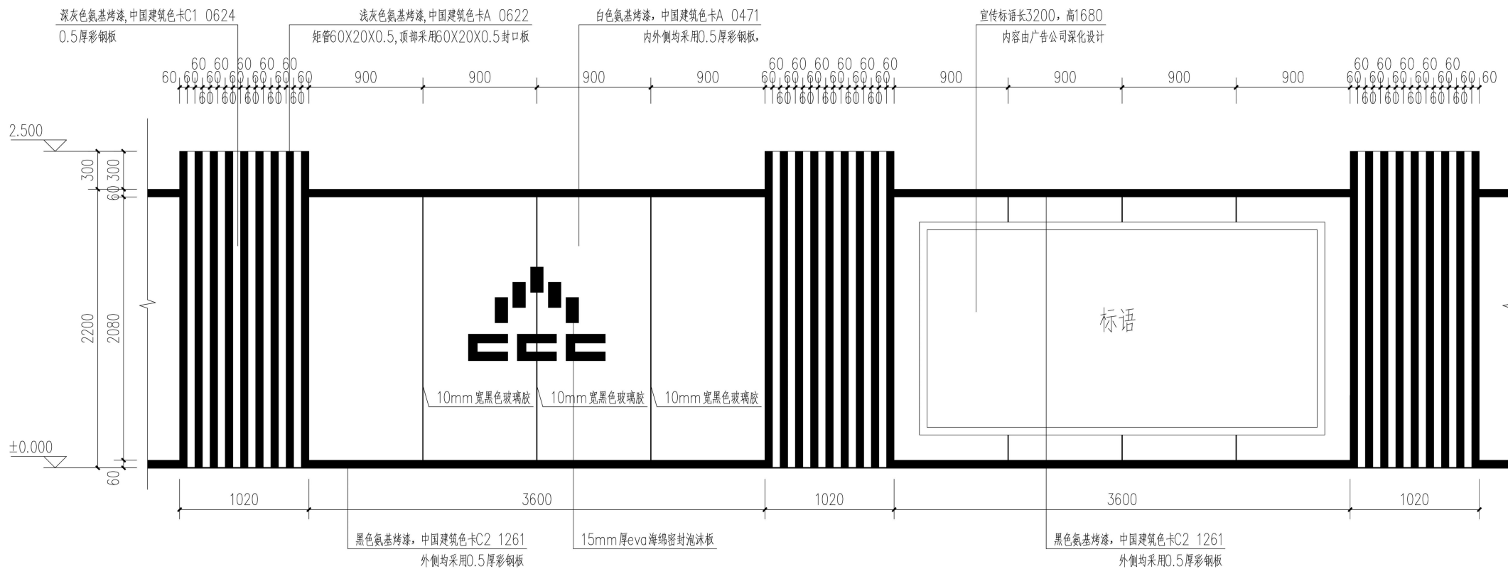
围挡立面图
