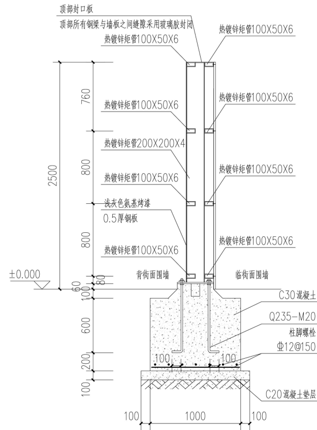
1-1剖面图
