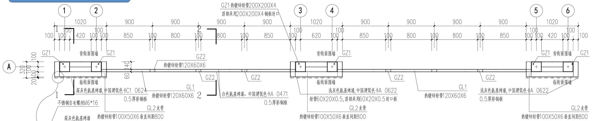
围挡平面图
